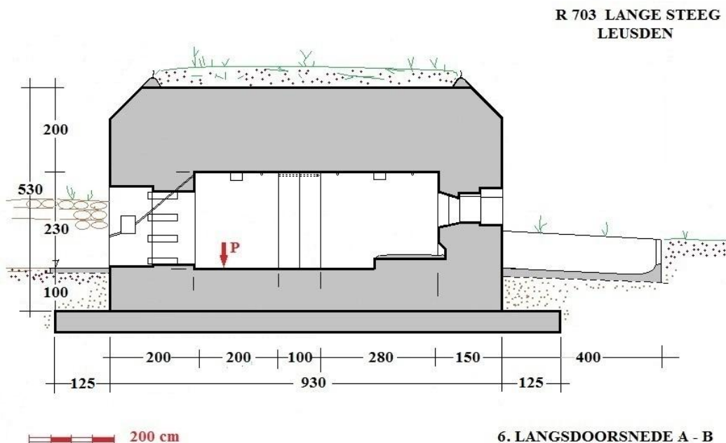
doorsnede R703 met rechts de mondingsgaskuil
