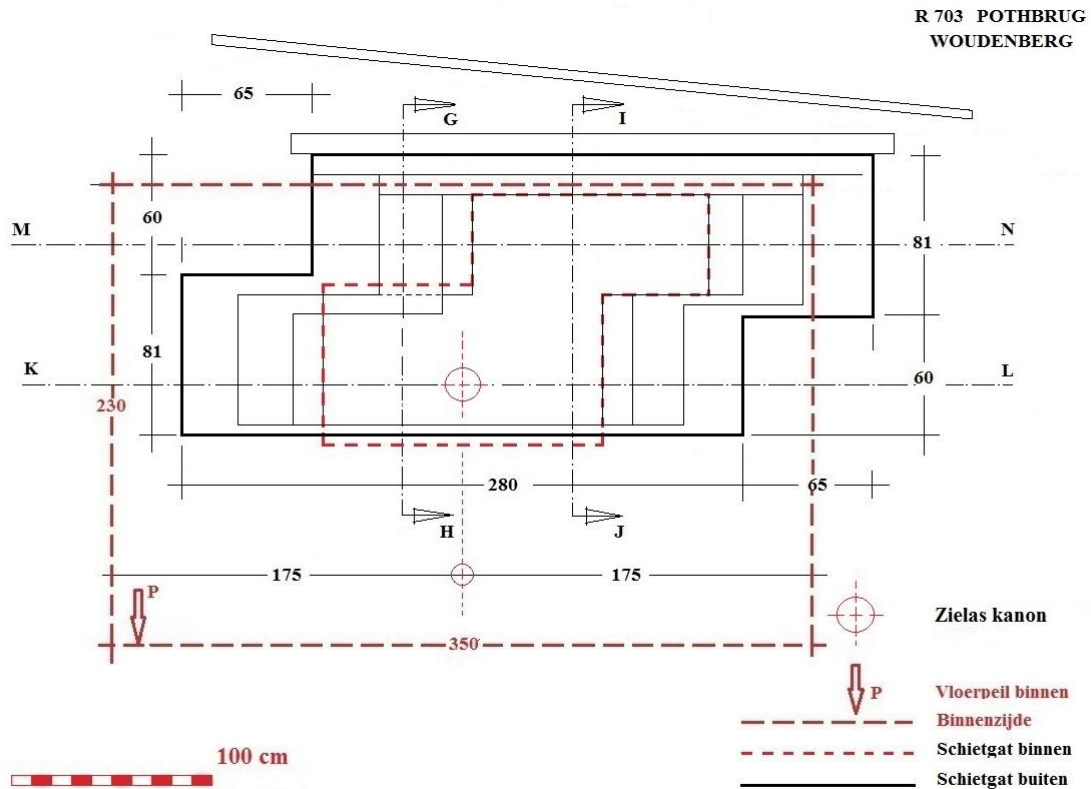
8. BUITENAANZICHT SCHIETGAT
