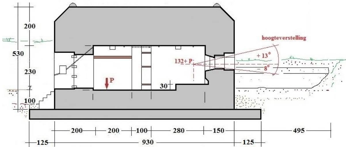
6. LANGSDOORSNEDE A - B
