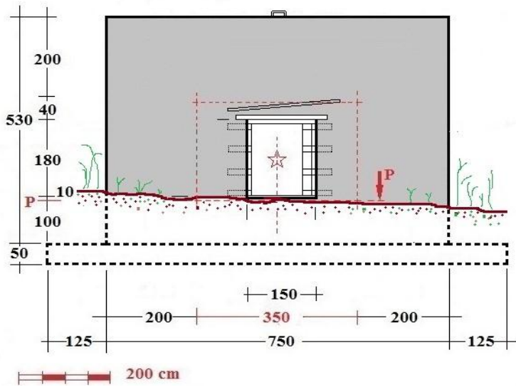
3. ACHTERAANZICHT
